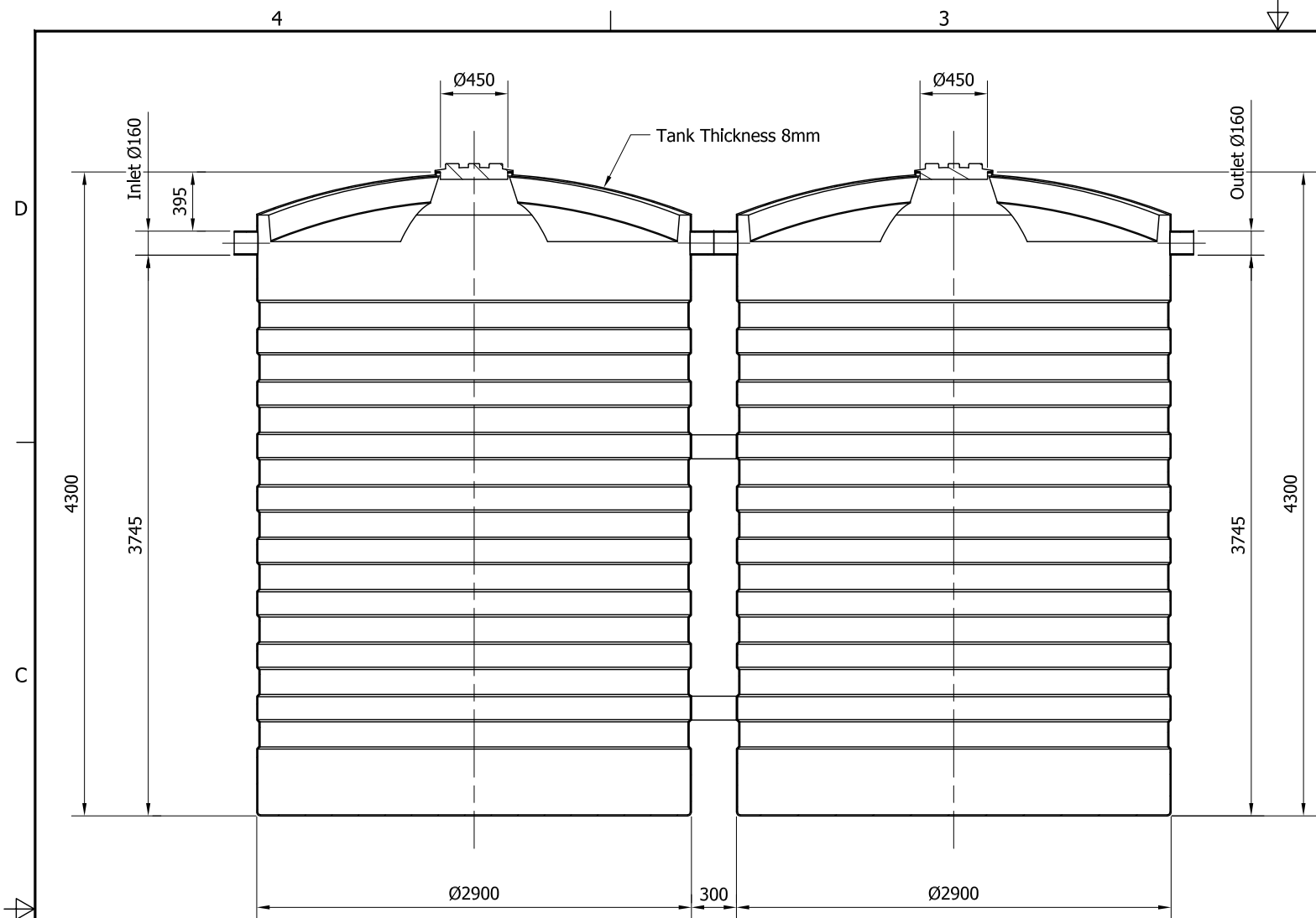
SECTION A-A
